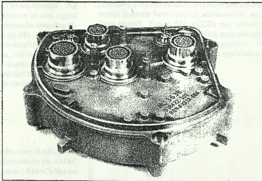
Figure 27. MC3638 ICU.
